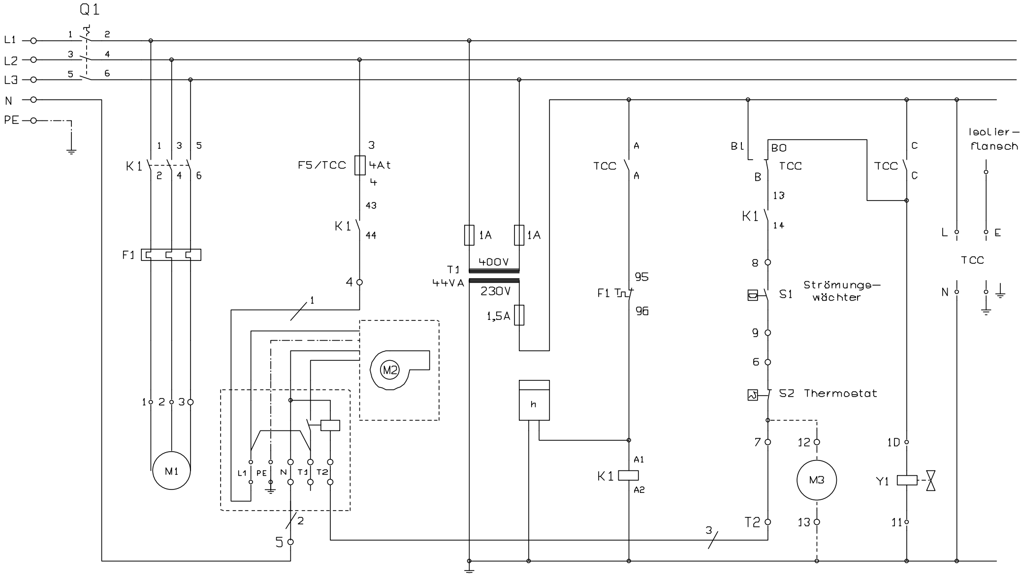
Brenner Ansteuerung
